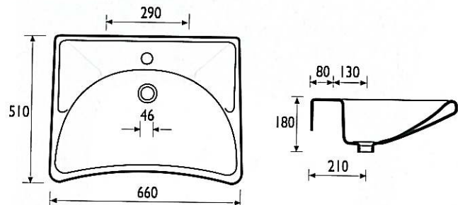
Réf. LA 00 200 FIXATION PAR BOULONS (FOURNIS)
