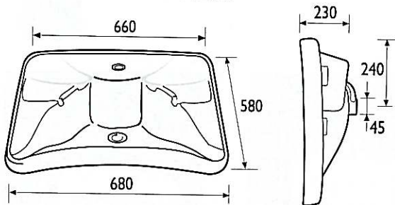
Réf. LA 00 100 FIXATION SUR CONSOLE (FOURNIE EN OPTION)
