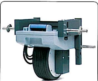
Base motrice du viamobil® Bandage plein increvable, système de ressort automatique pour traction constante, levage automatique de la roue.
