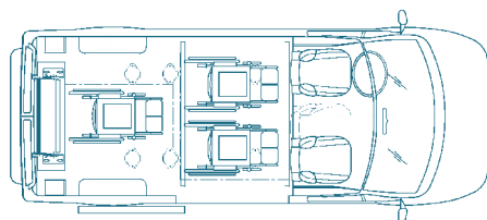
Version 3 fauteuils roulants
