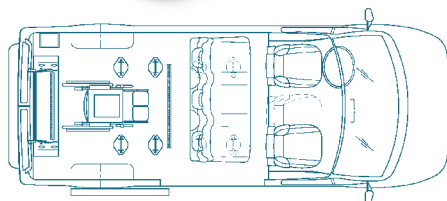
Version 1 fauteuil roulant
