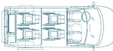
Version 4 fauteuils roulants
