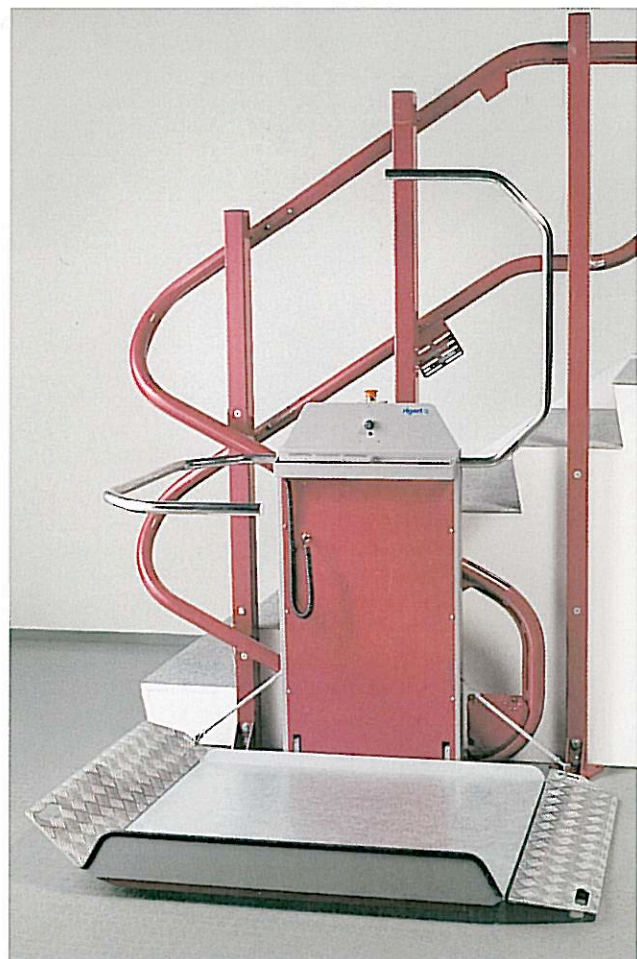
Le TLG-PEGASUS à l'arrêt inférieur avec bras de sécurité relevé, prêt pour l'utilisation.
