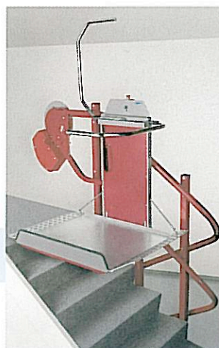
Le TLG-PEGASUS à l'arrêt supérieur, plateforme abaissée.
