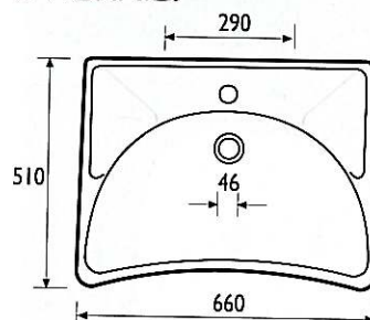
Réf. LA 00 200 FIXATION PAR BOULONS (FOURNIS)
