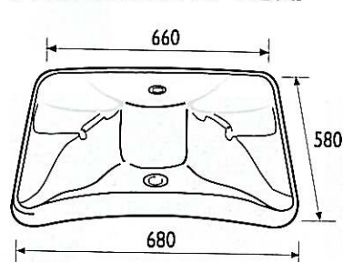
Réf. LA 00 100 FIXATION SUR CONSOLE (FOURNIE EN OPTION)
