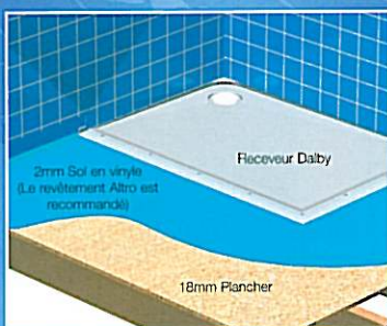
▲ Le Dalby se loge dans l'épaisseur des planchers de 18 mm et il n'est donc plus nécessaire d'augmenter l'épaisseur du reste du sol.
