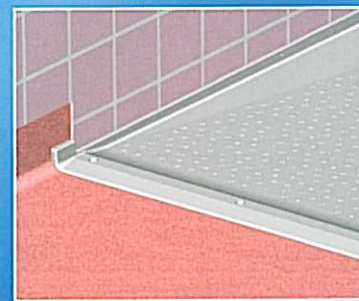
▲ Feuillure spécialement conçue pour fixer le matériau de revêtement de sol au mur pour en permettre l'étanchéité avec un produit de type mastic ou silicone.
